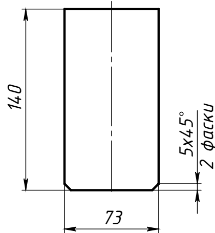
Поз.3 (Ребро среднее)
