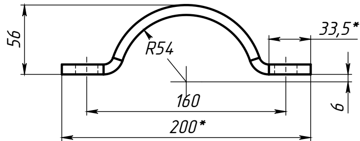
Поз.4 (Полухомут)
