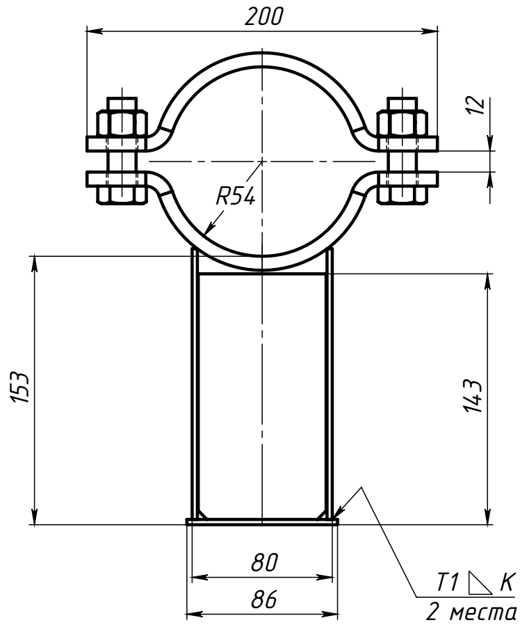
Поз.4 (Полухомут)
