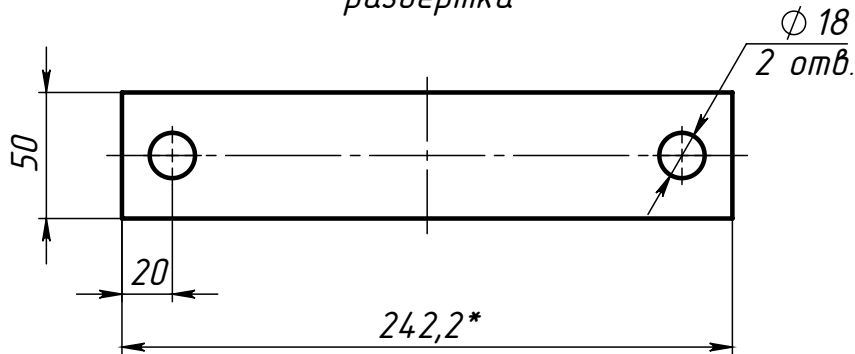
Поз.4 (Полухомут) развертка
